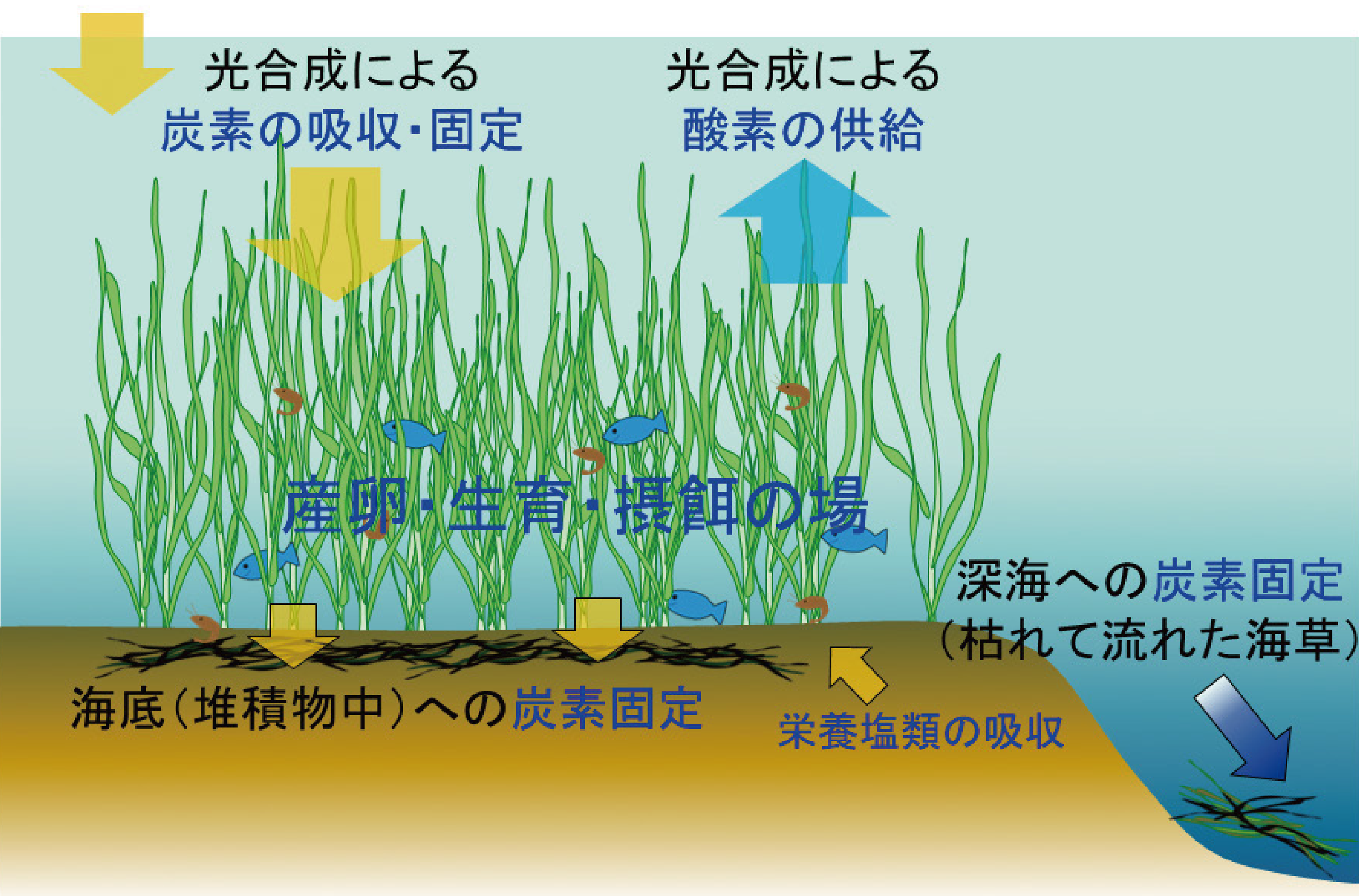
藻場の機能
